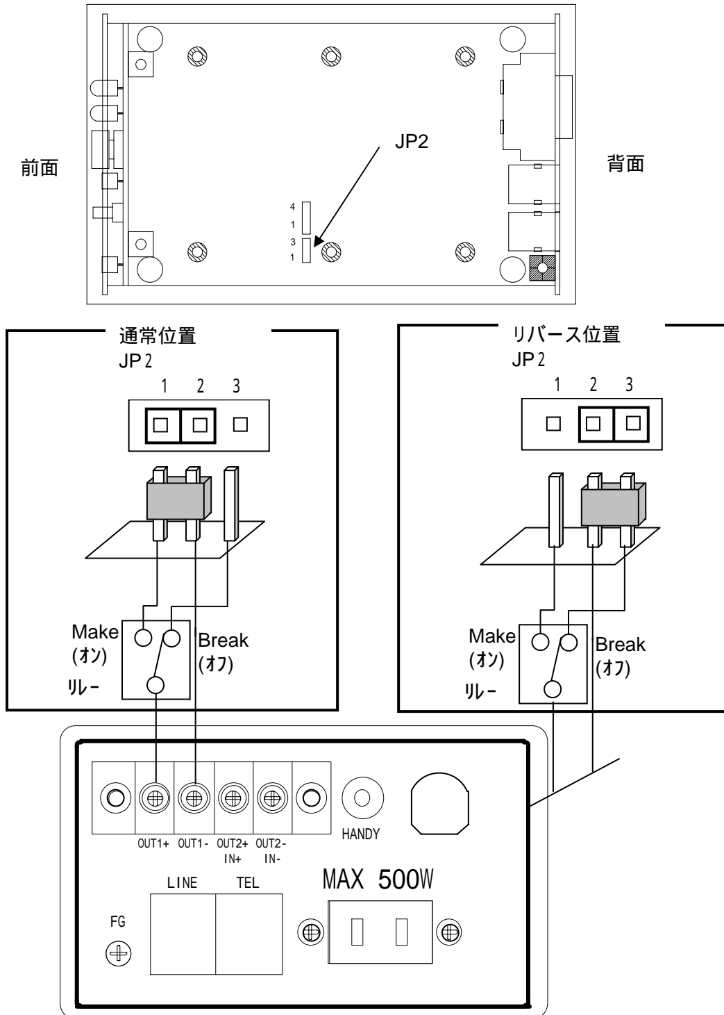
図8 - 2 リレー接点出力回路
